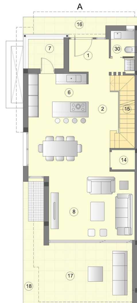
PLANTA BAJA
